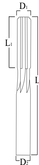
Диаграмма Развертки
