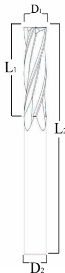
Диаграмма Фрезы
