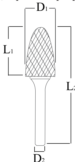
Диаграмма Бор-Фрезы
